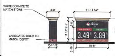
9 KROGER MONUMENT SIGN SCALE: NTS
